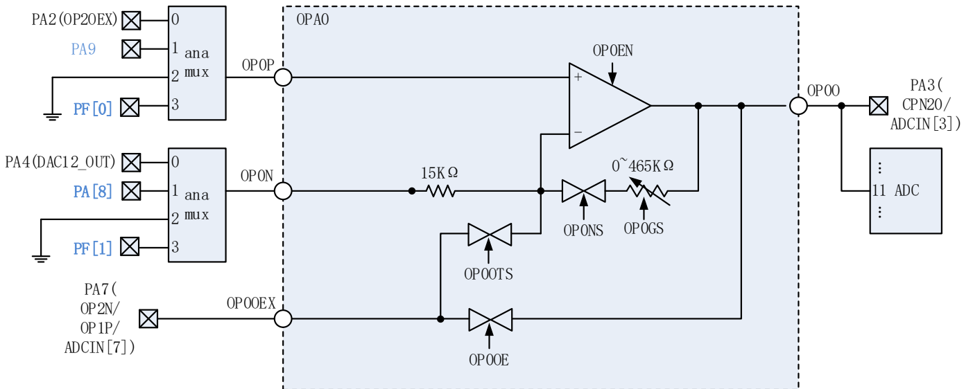
图 7. OPA0 内部结构和外部互联
