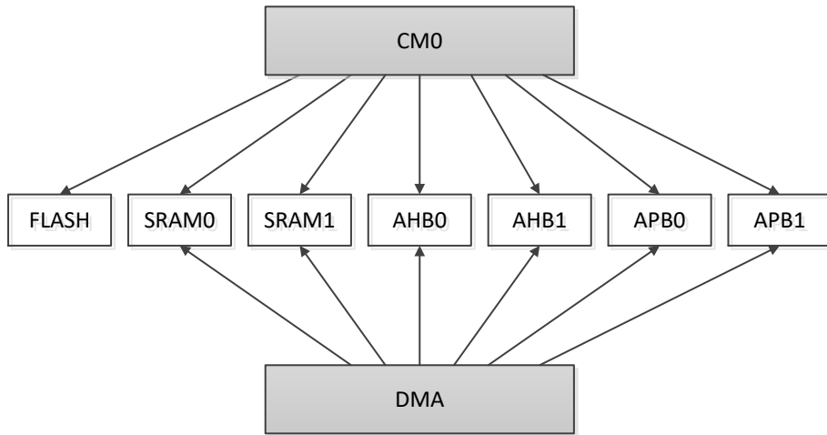
图 3. LCM32F038/X 总线矩阵
