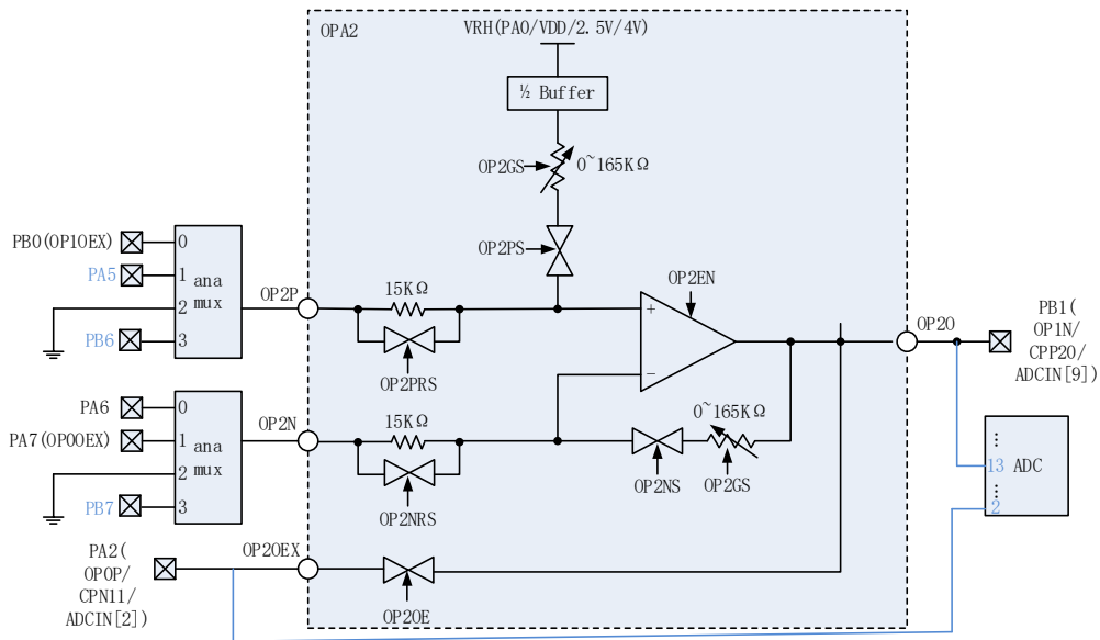
图 9. OPA2 内部结构和外部互联
