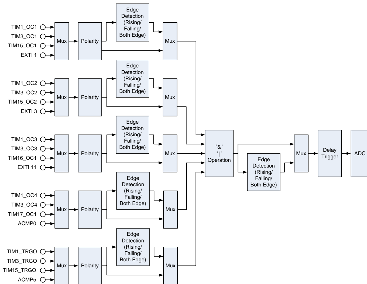
图 5. ADC 触发互联框图
