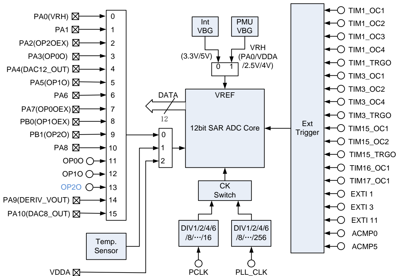
图 4. ADC 框图
