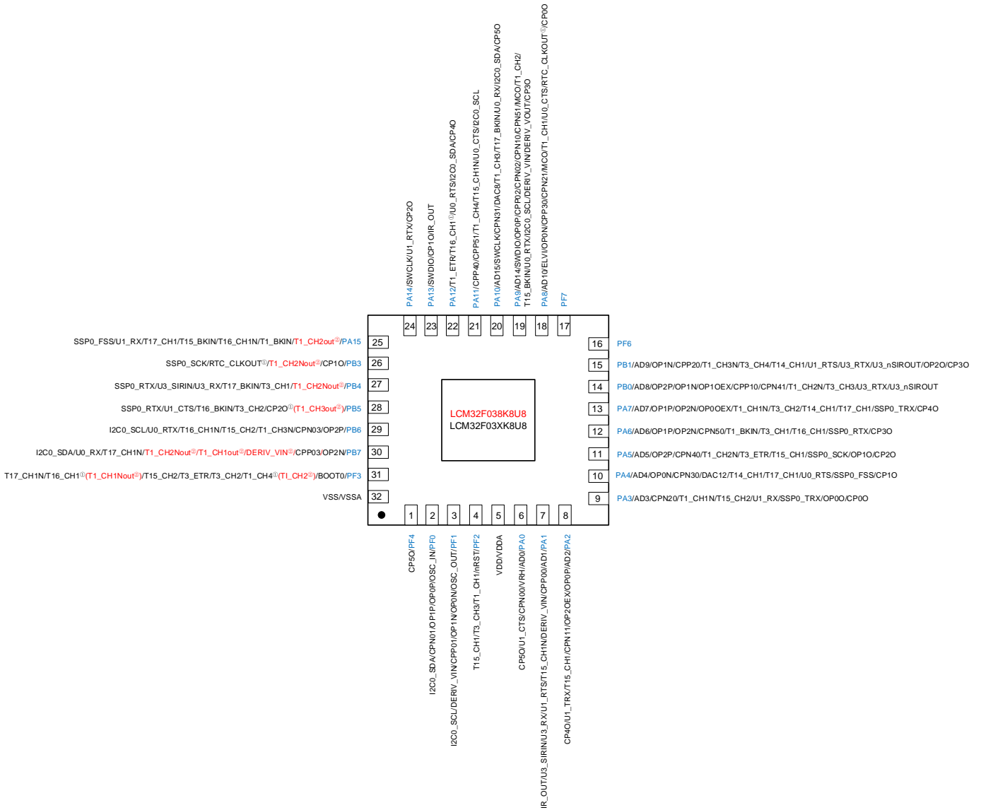
图 12. LCM32F038/XK8U8 QFN32 封装引脚排列
