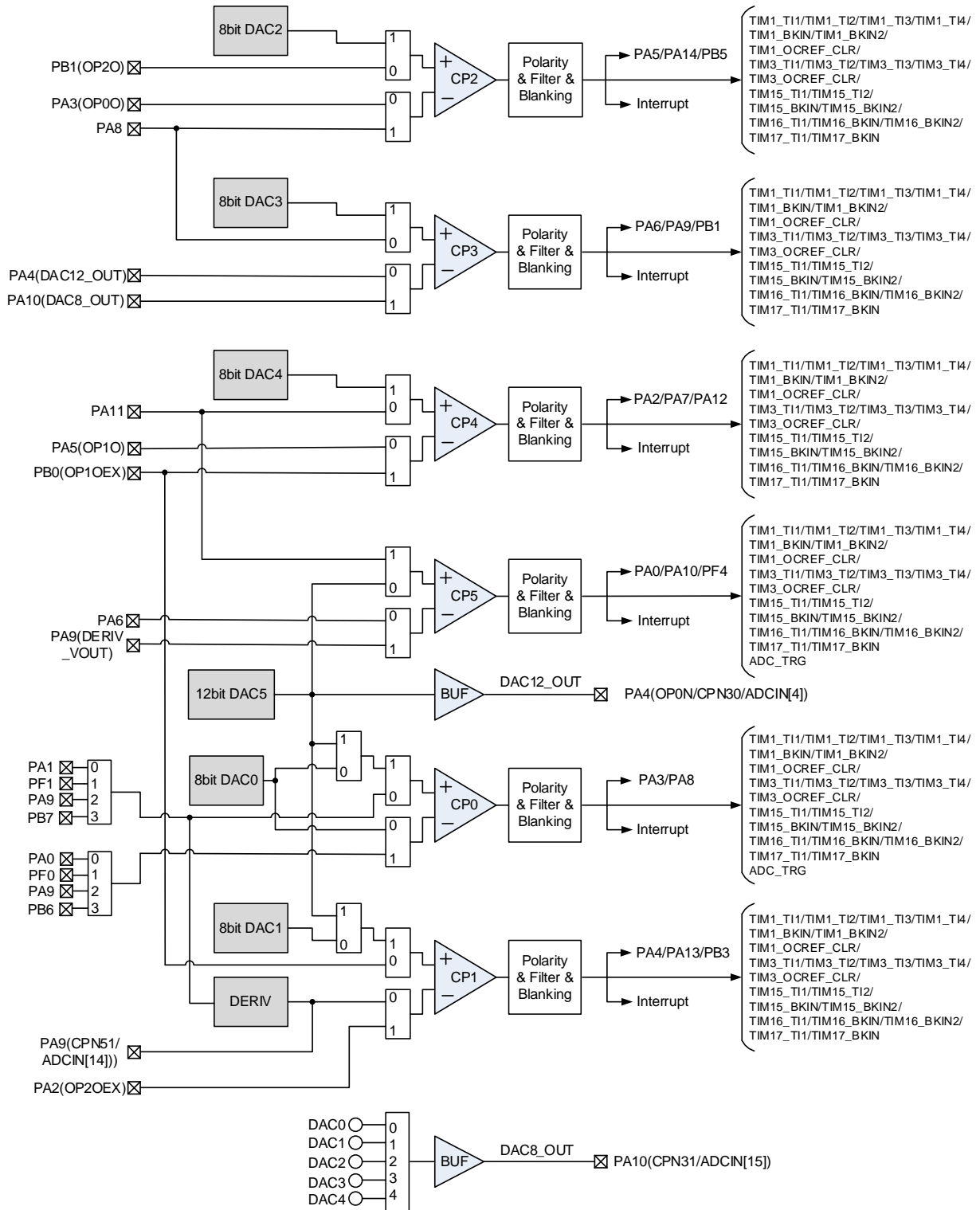
图 6. DAC 和 ACMP 互联
