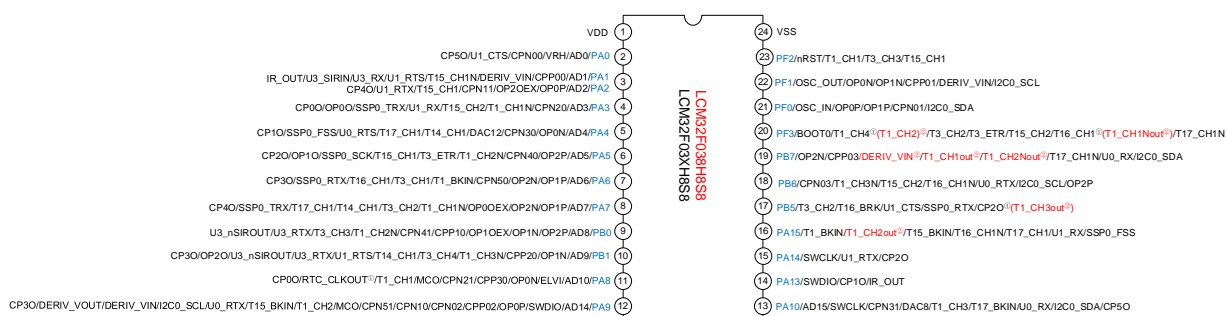
图 13. LCM32F038/XH8S8 SSOP24 封装引脚排列
