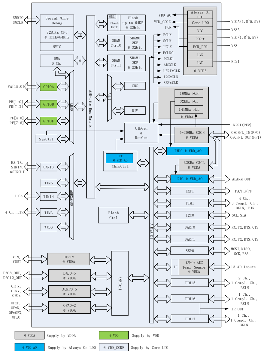
图 1. LCM32F038/X 模块框图
