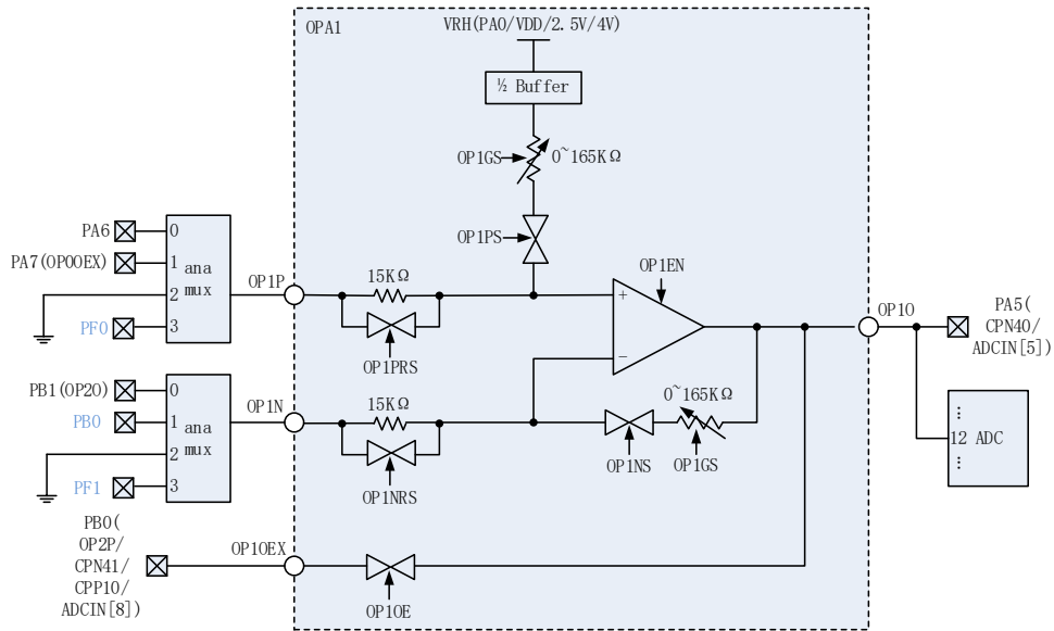
图 8. OPA1 内部结构和外部互联
