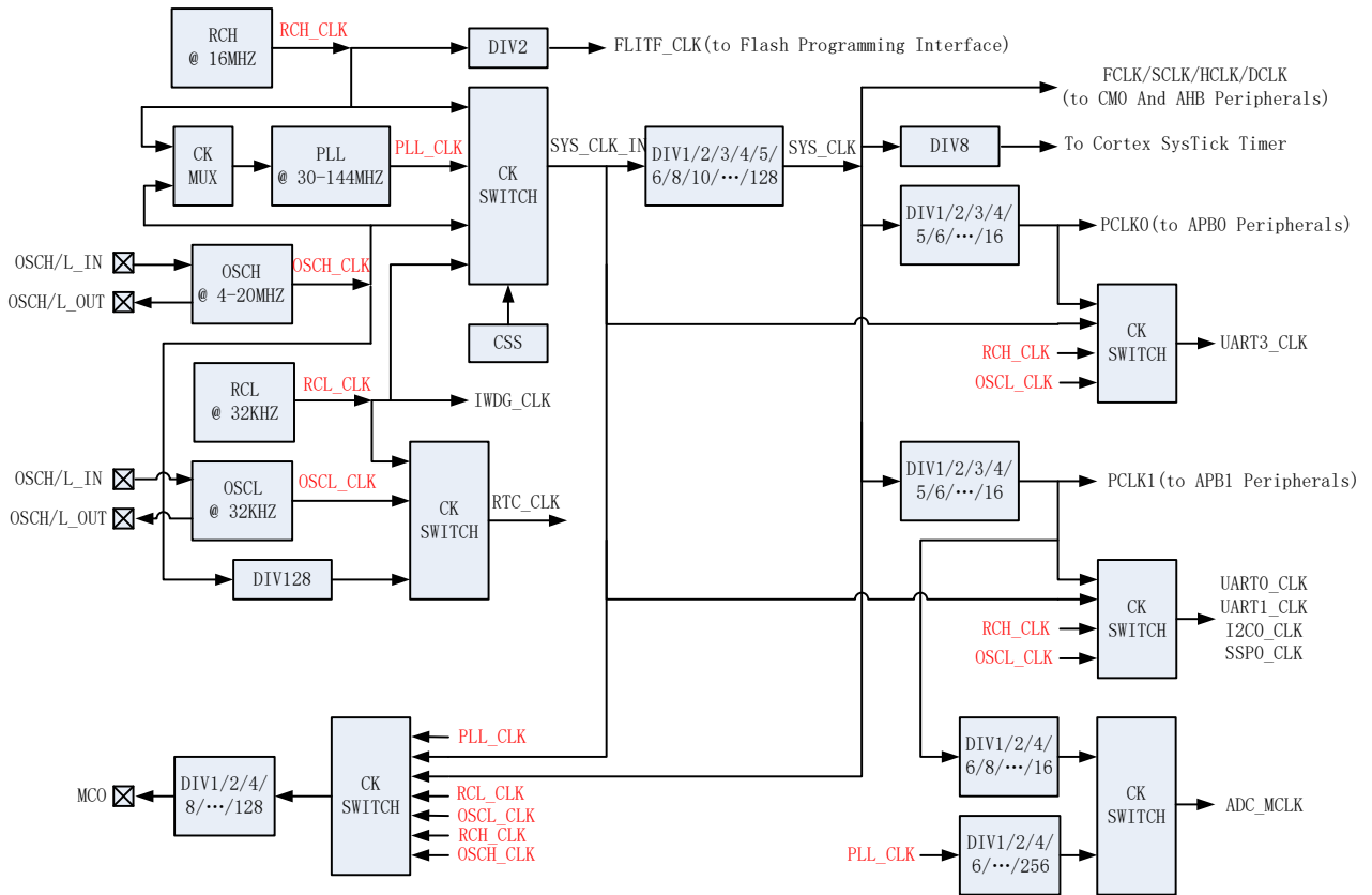
图 2. LCM32F038/X 时钟树
