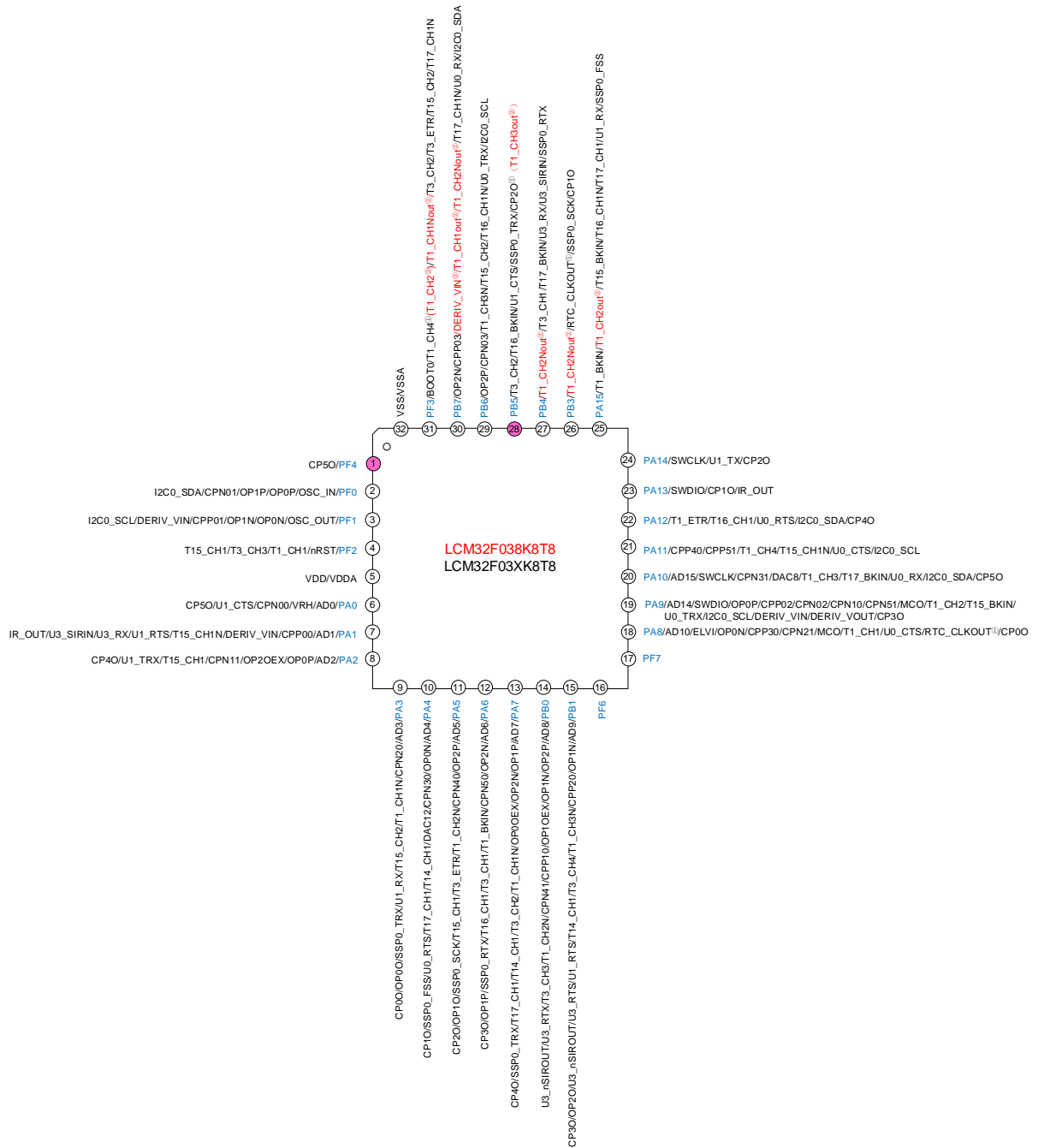
图 11. LCM32F038/XK8T8 LQFP32 封装引脚排列
